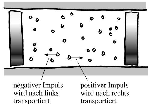
Abb. 3. Ein Teilchenstrom von links nach rechts und einer von rechts nach links, aber nur ein Impulsstrom von links nach rechts.
