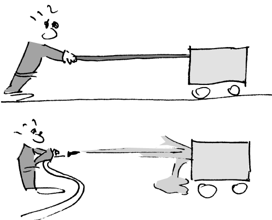
Abb. 2. Für die beiden Impulstransporte sind unterschiedliche Sprechweisen üblich. Oben: „Auf den Wagen wirkt eine Kraft“. Unten: „Das Wasser transportiert Impuls“.
